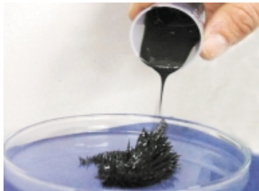
Cambio de la viscosidad de un fluido magnetoreológico ante un campo magnético
