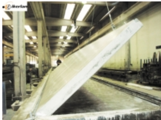
Sensores de fibra óptica embebidos en la estructura de hormigón, IKERLAN
