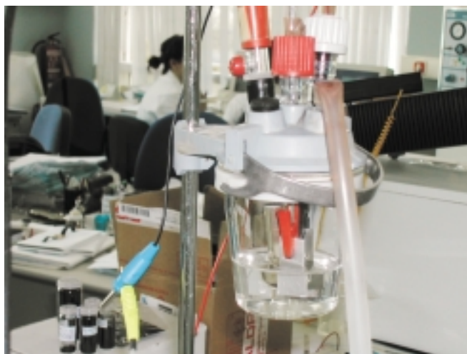
Preparación de un film electroactivo por electropolimerización (EAP) para su empleo en Fotovoltaicos, CIDETEC
